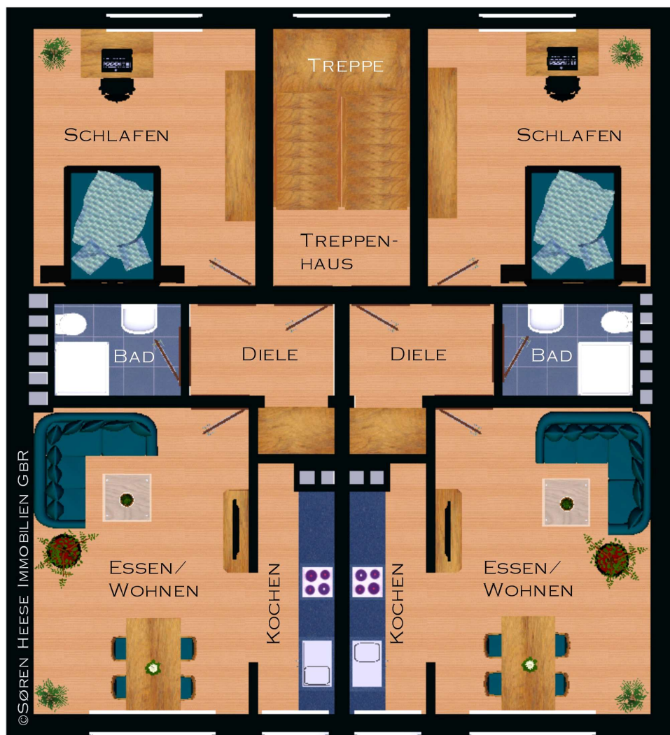
- DAS 1. OBERGESCHOSS -
