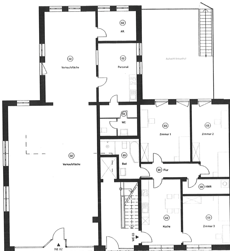
- DAS ERDGESCHOSS -
