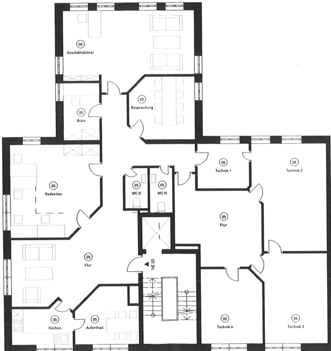
- DAS 2. OBERGESCHOSS -
